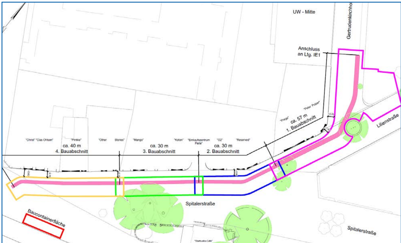
Lageplan der Baumaßnahme Spitalerstraße
